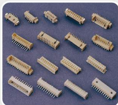
1.25mm (.049") ■ Housing : JS-1146 Wafer : JS-1147, JS-1147A(180°)-DIP JS-1147R(90°,DIP) JS-1147V(180°,SMT) JS-1147H(90°,SMT) Terminal : JS-1146-T ■ Poles : 02-15
