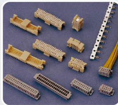
1.25mm (.049") ■ Housing : JS-1255 Wafer : JS-1256(SMT) Terminal : JS-1225-T / TG ■ Poles : 5*2-25*2
