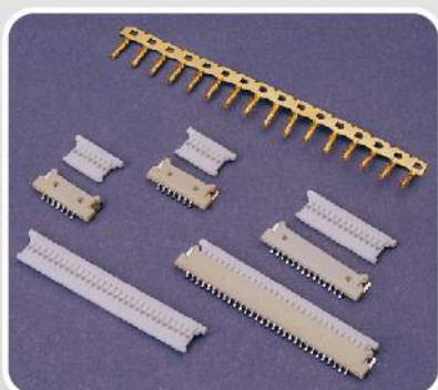
1.25mm (.049") ■ Housing : JS-1258 Wafer : JS-1259(SMT) Terminal : JS-1258-T / TG ■ Poles : 02-30
